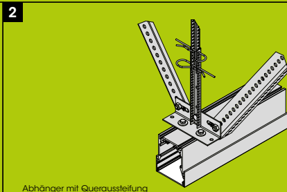
2 Abhänger mit Queraussteifung Hanger with lateral bracing Suspension avec renforcement transversal
