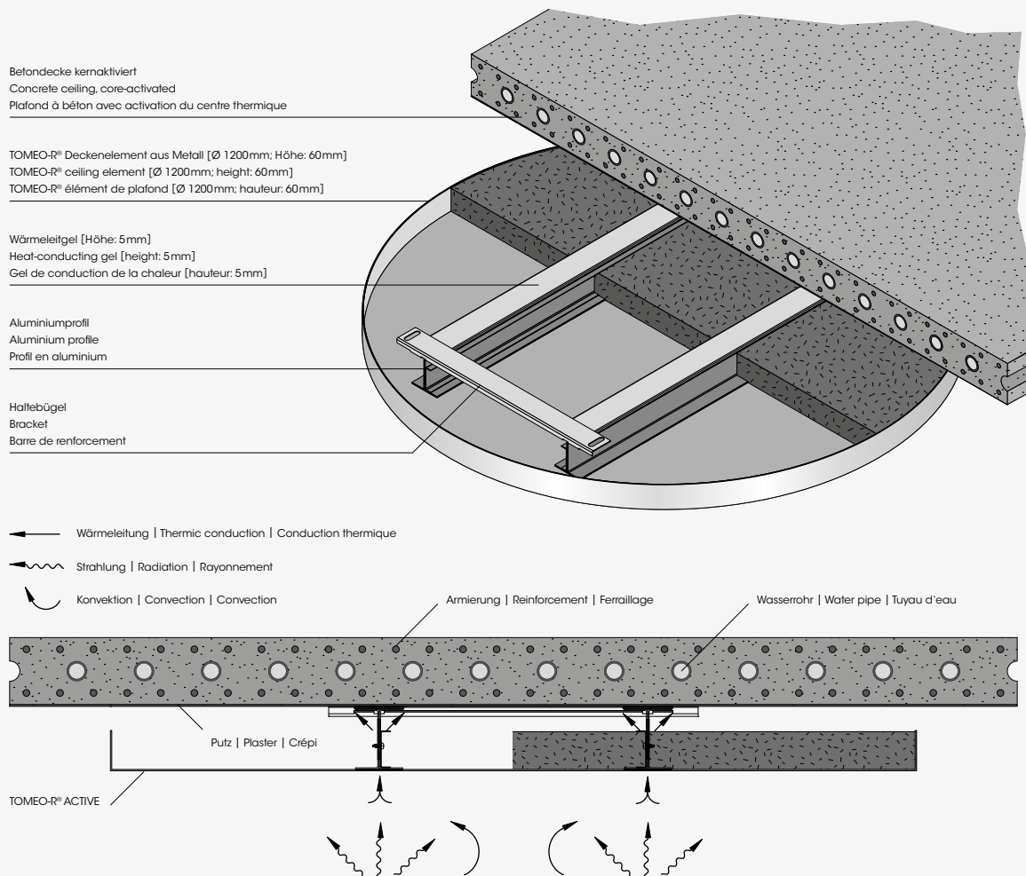
Funktionsweise TOMEO®-R und LUMEO®-R ACTIVE | Functioning of TOMEO®-R and LUMEO®-R ACTIVE | Fonctionnement TOMEO®-R et LUMEO®-R ACTIVE
